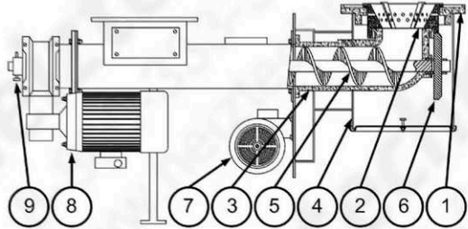
Поворотная ретортная горелка
