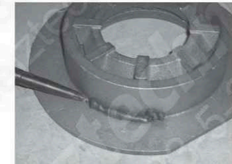
Нанесение герметика между короной и корпусом горелки на неповоротной ретортной горелки
