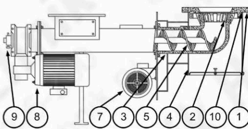
Неповоротная ретортная горелка
